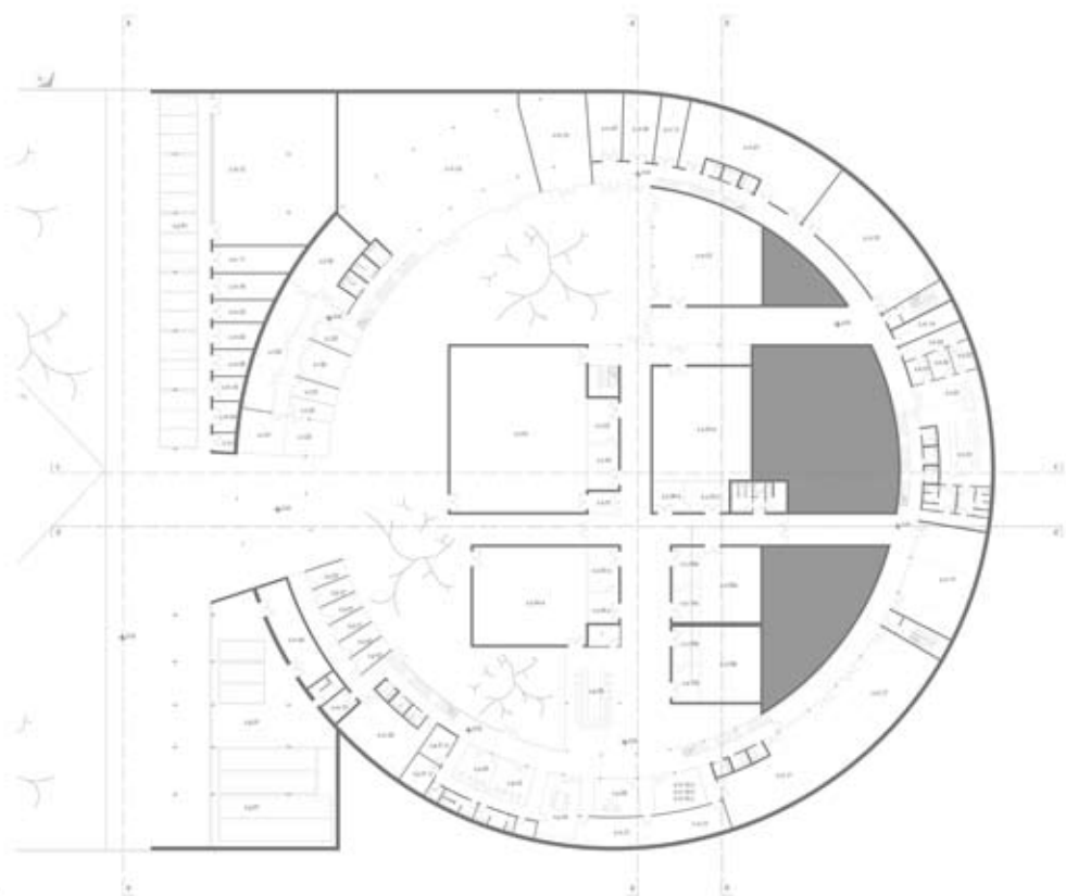
PRESEK C-C
